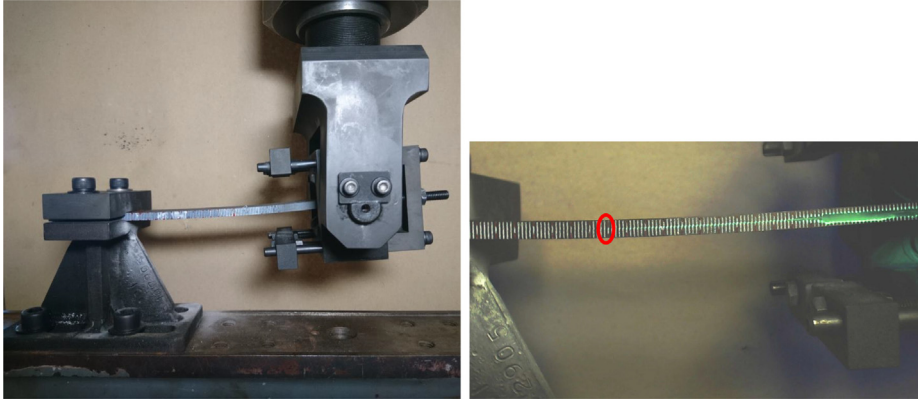
(a) ELS test device
