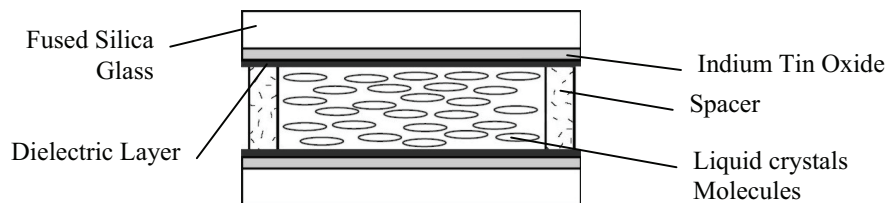
4.a : Maximal retardance V=0
