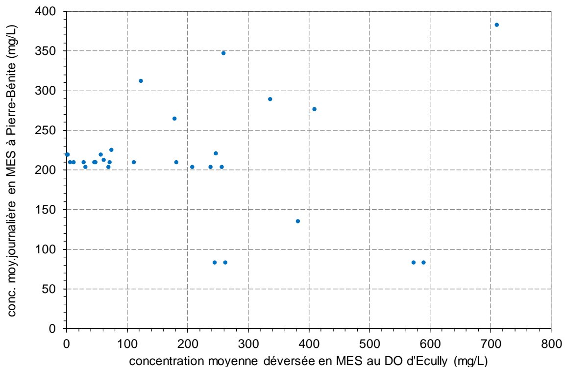
Figure 4 : Concentrations moyennes journalières en MES à la STEU de Pierre-Bénite et concentrations moyennes déversées en MES mesurées au DO d'Ecully, 30 déversements, année 2004.
