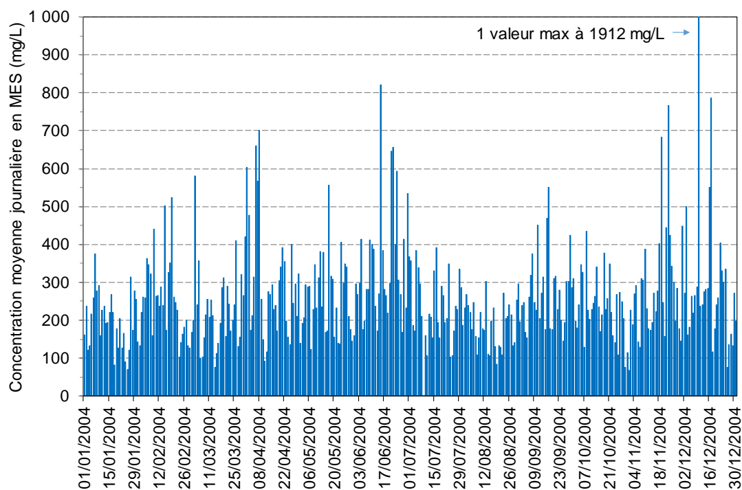
Figure 3 : Concentrations moyennes journalières en MES à l'entrée de la STEU de Pierre-Bénite, année 2004 complète.
