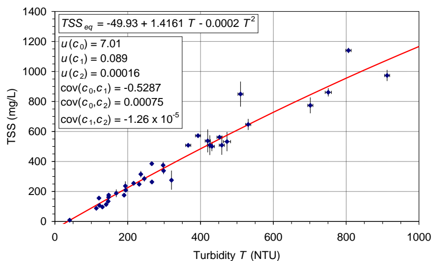
Figure 1 : Relation turbidité-MES, DO Valvert, Ecully (source : Bertrand-Krajewski et al. , 2007).
