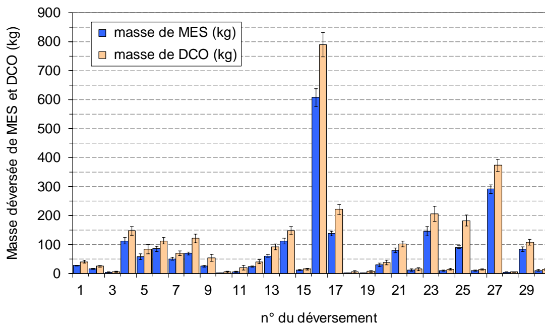
Figure 2 : Masses déversées de MES et DCO par les 30 déversements mesurés en 2004 au DO d'Ecully (source : Bertrand-Krajewski et al. , 2007).
