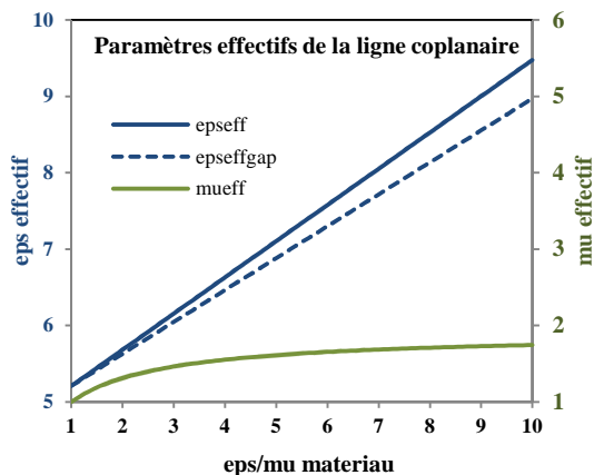
Fig. 2: Evolution des paramètres effectifs de la cellule de mesure en fonction de la permittivité et de la perméabilité du matériau. h_{\text{mat}}=2\text{mm} ; h_{\text{sub}}=3.2\text{mm} ; \epsilon_{\text{sub}}=9.6 ; \text{gap}=50\mu\text{m}
