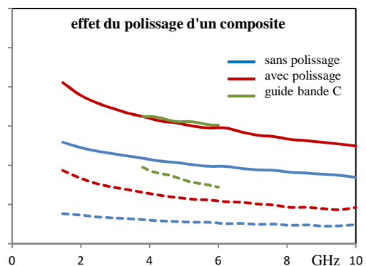
Fig. 8. Comparaison de la permittivité mesurée d'un même échantillon sur ligne coplanaire et en guide d'onde rectangulaire bande C. Influence de l'état de surface des échantillons.
