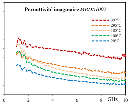
Fig. 10: Evolution de la permittivité réelle et imaginaire d'un matériau dispersif pour des températures de 20°C à 400°C.
