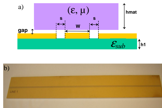
Fig. 1: (a) Dessin de la section transverse de la ligne coplanaire. (b) ligne réalisée 300 x 40 x 5 mm 3 , W=1075 \mu\text{m} , S= 535 \mu\text{m} .
