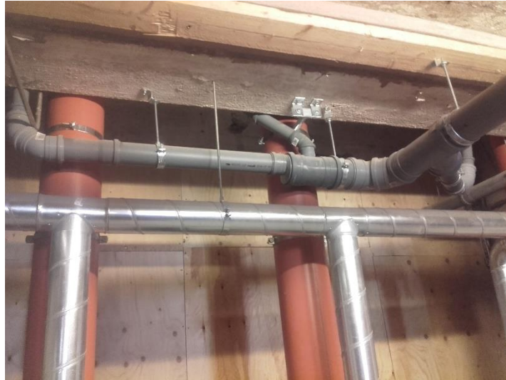
Figure 6 : Réseau de collecte d'urine (PVC), de chute des matières fécales (rouge) et de ventilation des cuves de collecte des matières fécale (argenté) à Tampere - Finlande
