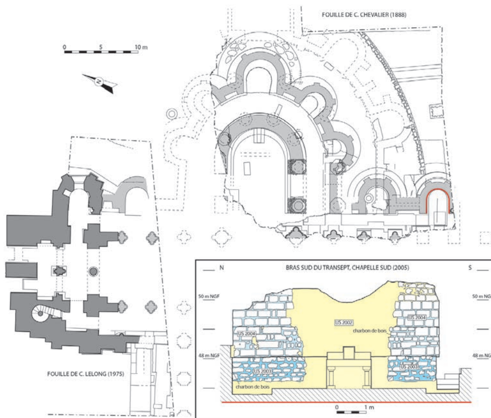
Fig. 4. Tours (Indre-et-Loire), Saint-Martin, plan des parties orientales d'après les fouilles du chevet (C. Chevalier, Les fouilles... , 1888, pl. h. t.) et du bras nord du transept (C. Lelong, Le transept... , 1975, p. 114) et relevé développé de la chapelle méridionale du bras sud du transept (relevés et DAO : P. Martin, 2005).
