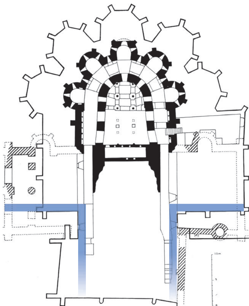
Fig. 8. Orléans (Loiret), Saint-Aignan, plan des fouilles, d'après F. Lesueur ( Bulletin monumental , 1957, p. 199). En bleu figure la position des murs occidentaux du transept et la largeur de la nef selon les nouvelles observations exposées dans cet article.
