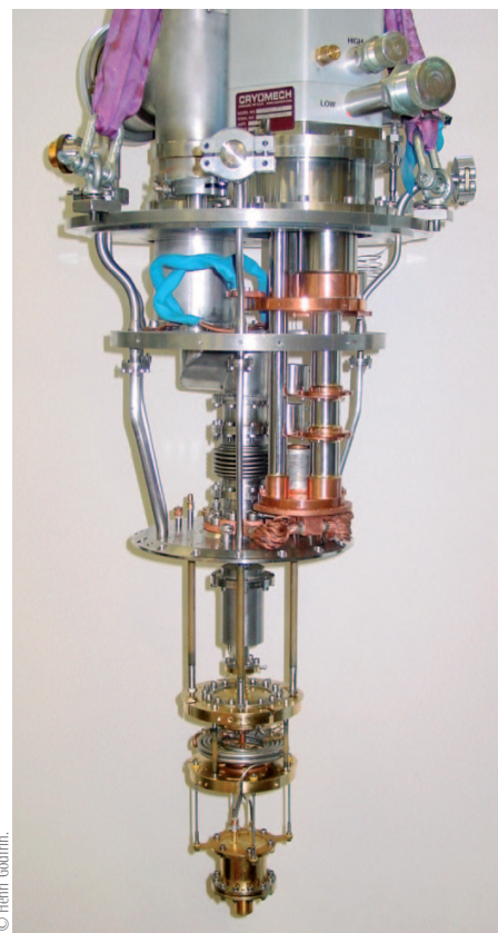
3. Réfrigérateur à dilution ^3\text{He}-^4\text{He} permettant d'atteindre des températures de quelques millièmes de degré au-dessus du zéro absolu (Collaboration CNRS-Institut Néel/L'Air Liquide).
