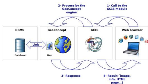
Fig.2:architecture du GCIS, serveur cartographique
