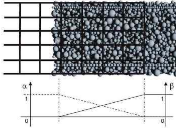
Figure 2. Zone de recouvrement et paramètres de recouvrement
