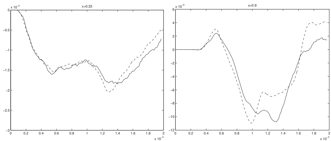
(c) Déplacement d'un ED à 0.33m de l'impact (d) Comparaison du déplacement d'un nœud EF et d'un ED
