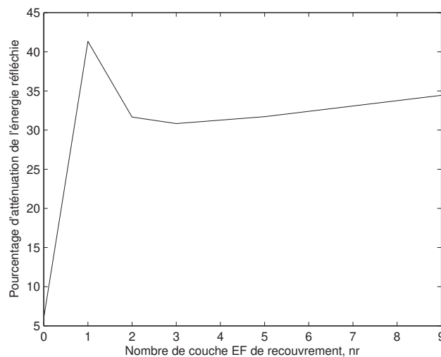
Figure 4. Influence de la diagonalisation en fonction de la taille de la zone de recouvrement sur le pourcentage d'atténuation de l'énergie réfléchi
