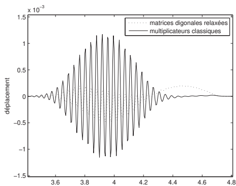
(b) Onde HF réfléchi
