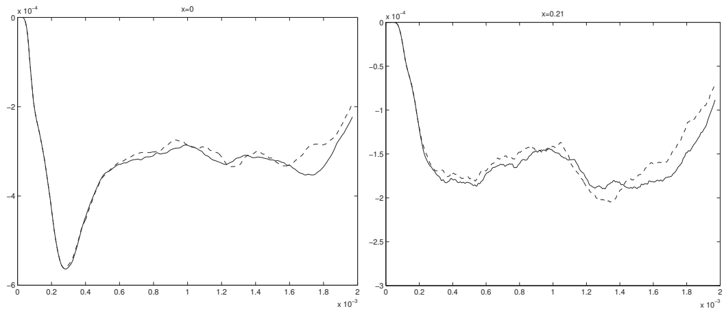
(a) Déplacement d'ED sous l'impact - (b) Déplacement d'un ED à 0.21m de l'impact
