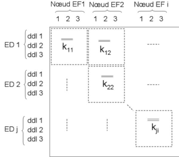
Figure 3. Organisation des matrices de couplage en sous-matrices
