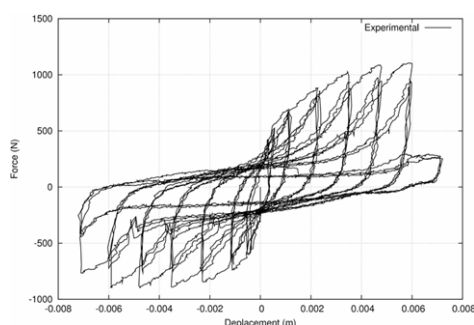
Figure 8. Exemple de comportement hystérique force-déplacement
