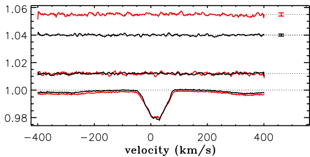
Fig. B.27. LSD profiles for Par 1736 (no magnetic detection).
