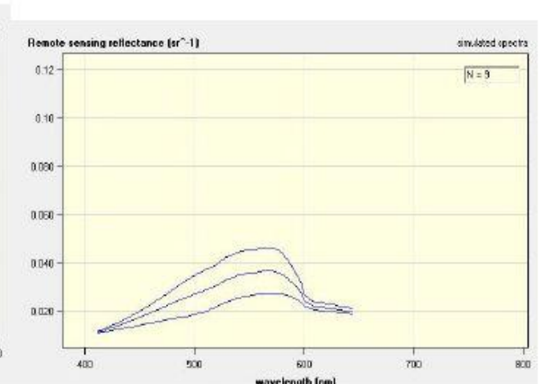
(d) SeaWiFS
