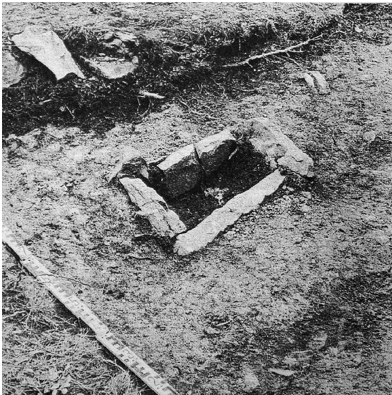
Figure 11 : Altenberg, « four d'essai », site 24, aire de travail III, 1972, dans DAHM, Cl., LOBBEDEY, U., WEISGERBER, G., Der Altenberg. Bergwerk und Siedlung aus dem 13. Jahrhundert im Siegerland , Dr. Rudolf Habelt GMBH, Bonn, 1998, band 1, p. 95.
