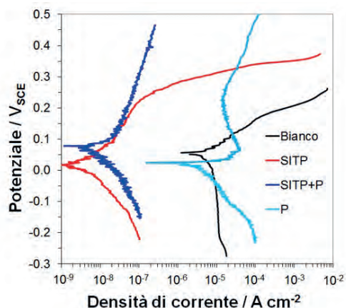
Fig. 2 - Curve di polarizzazione registrate su elettrodi di bronzo dopo 20 giorni di immersione in ARX10, in assenza di inibitori e in presenza di SITP saturo, SITP saturo + 10 -2 M P e in presenza di 10 -2 M P.
