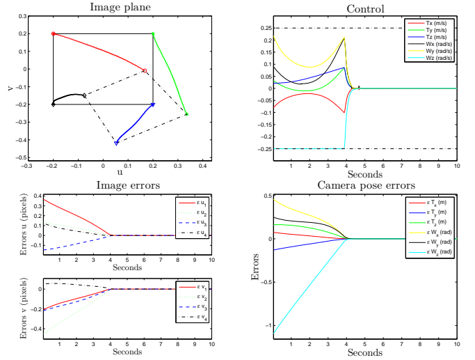
Fig. 13. N_p = 5 and Q = I
