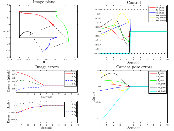
Fig. 12. N_p = 1 and Q = I
