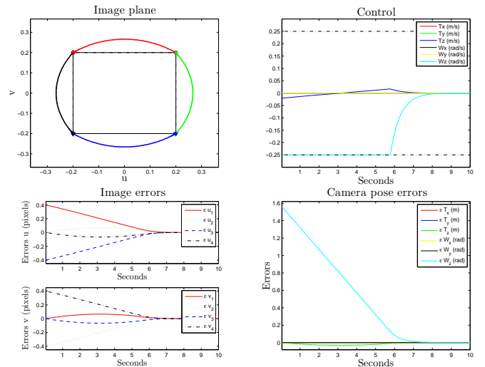
Fig. 8. N_p = 20 and Q = I
