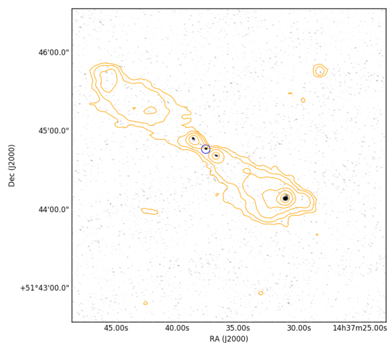
A.1. 32 ILTJ143735.74+514434.3 † ROBUST: -0.5
