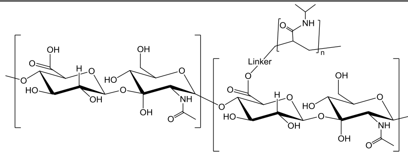
HA-g-PNIPAAm Hyaluronic acid-g-poly(NIPAAm)
