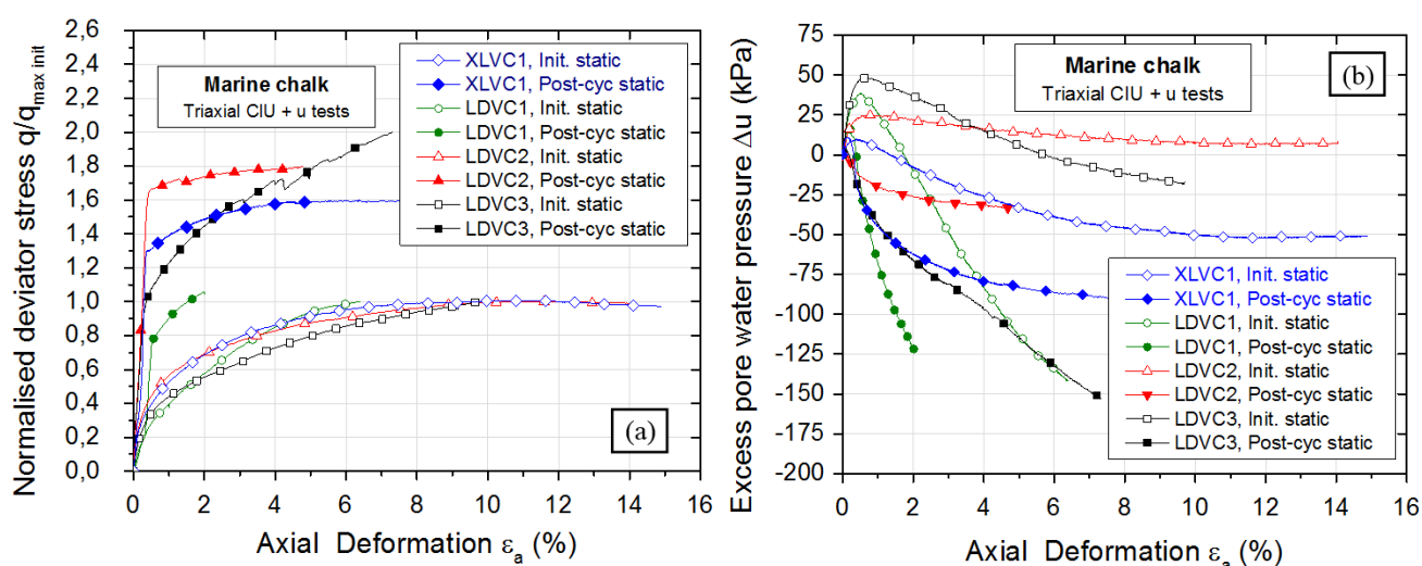
Figure 7. Effet du chargement cyclique sur le comportement statique post-cyclique : (a) déviateur des contraintes normalisées ; (b) évolution des surpressions interstitielles
