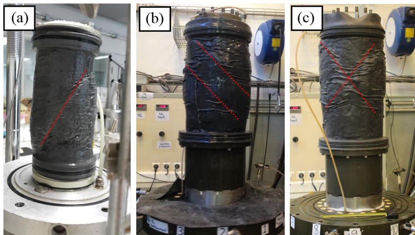
Figure 5. Vue des éprouvettes après l'essai de cisaillement statique : (a) VC ( \varnothing 100 mm) ; (b) LDVC ( \varnothing 300 mm) ; (c) XLVC ( \varnothing 300 mm)
