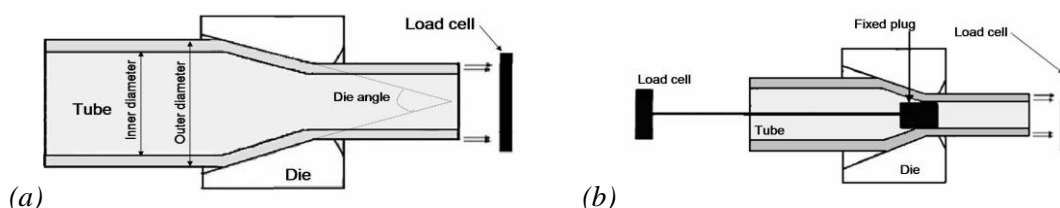
FIG. 1 – Schéma des bancs d'étréage : (a) à creux, (b) sur olive.
