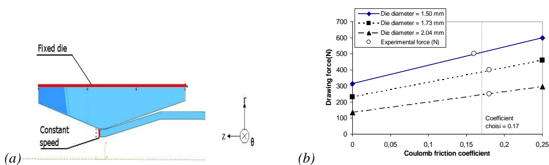
FIG. 3 – Étirage à creux : (a) Conditions aux limites, (b) Identification du coefficient de frottement.
