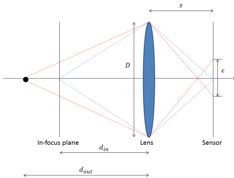
FIGURE 2 – Illustration du principe du DFD. Les rayons provenant du point flouté (point noir) convergent avant le capteur et s'étalent sur un disque de diamètre \epsilon .
