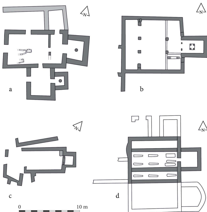
FIG. 8. — Comparación de las plantas de las iglesias de la Silla del Papa (a), San Pedro de Mérida (b), Ibahernando de Magasquilla de los Donaire (c) y Alcalá de los Gazules (d)
