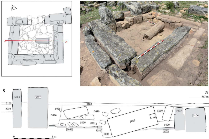
FIG. 4. — Vista desde el sureste y sección sur-norte del ábside, al final de la excavación y antes del levantamiento del soporte del altar
