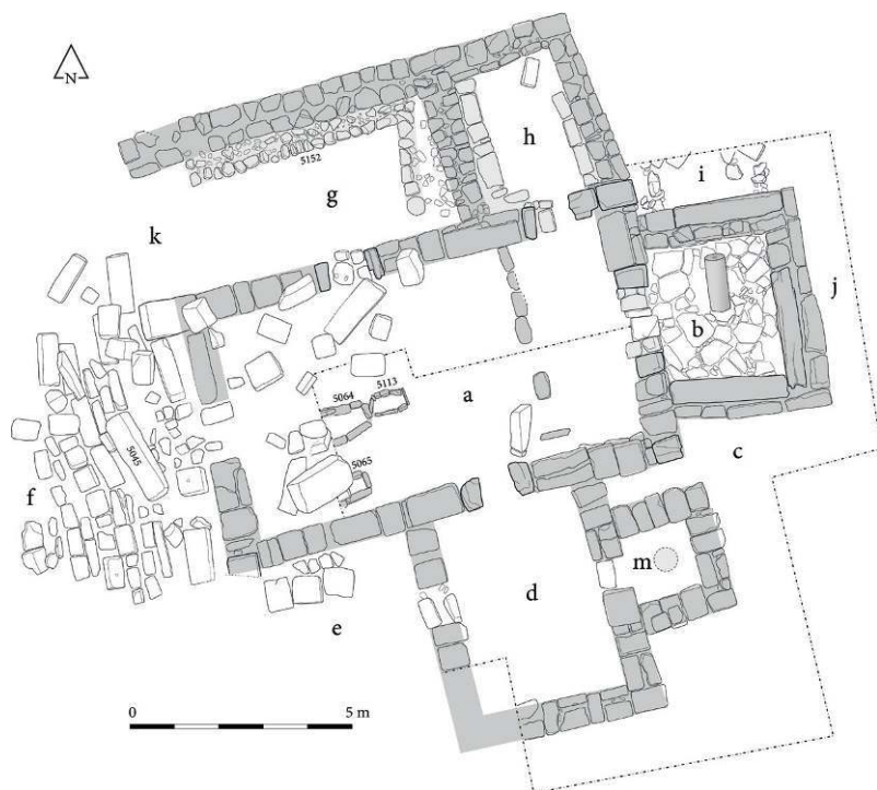
FIG. 3. — Plano de la iglesia de la Silla del Papa (sector D1)
