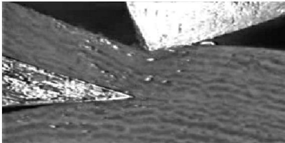
Figure 10.4.32. Efficacité de la barre de pression pour un placage de 2 mm.
