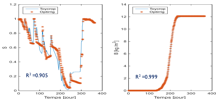
Fig. 3 – Simulation du taux d'humidité dans le sol et la production en Biomasse, stratégie pluviale, année 2011
