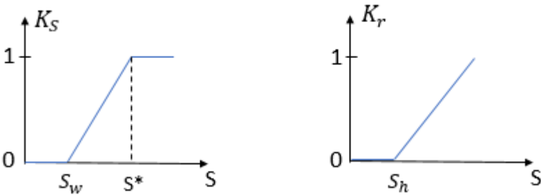
Fig. A.2– à gauche la fonction de limitation de la transpiration et à droite la fonction de limitation de l'évaporation
