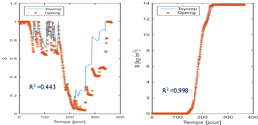
Fig. 1 – Simulation du taux d'humidité dans le sol et la production en Biomasse, stratégie pluviale, année 1996
