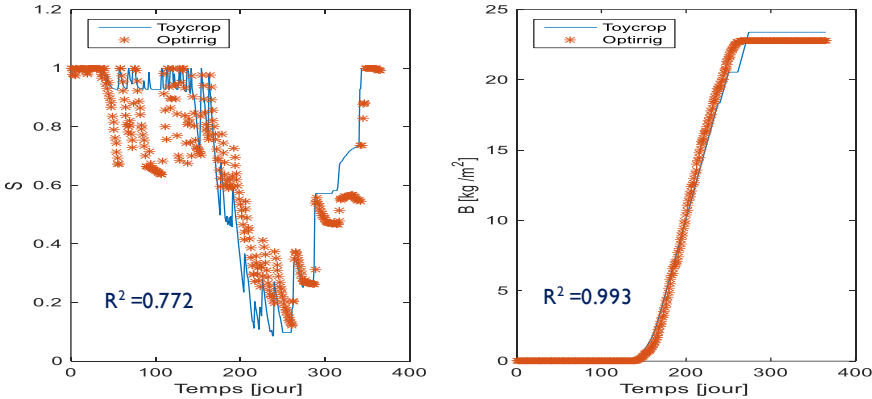
Fig. 2 – Simulation du taux d'humidité dans le sol et la production en Biomasse, stratégie tour d'eau, année 1996
