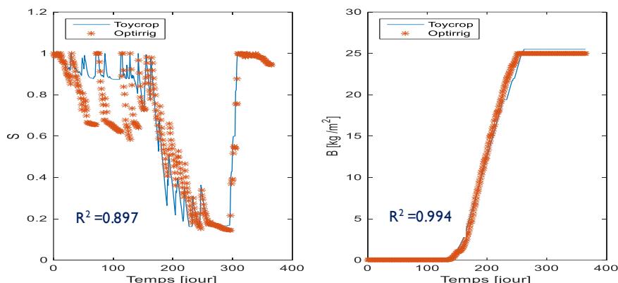
Fig. 4– Simulation du taux d'humidité dans le sol et la production en Biomasse, stratégie tour d'eau, année 2011
