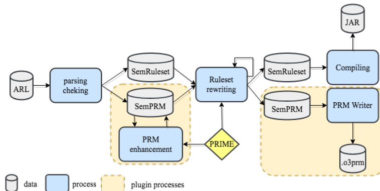
Figure 4. Utilisation du plugin PRIME dans la chaîne de compilation d’ODM
