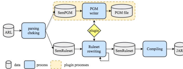
Figure 1. Représentation de la chaine de compilation d'ODM
