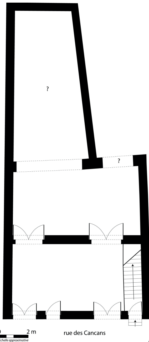
Fig. 12 : Proposition de restitution du plan du rez-de-chaussée. (Dessin : J. Foltran)
