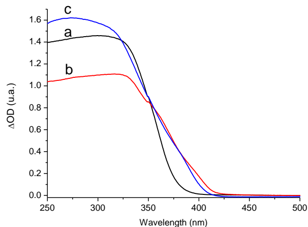
Fig.8 UV-vis spectra of (a) TiO 2 -P25, (b) TiO 2 -L and (c) TiO 2 -anatase.
