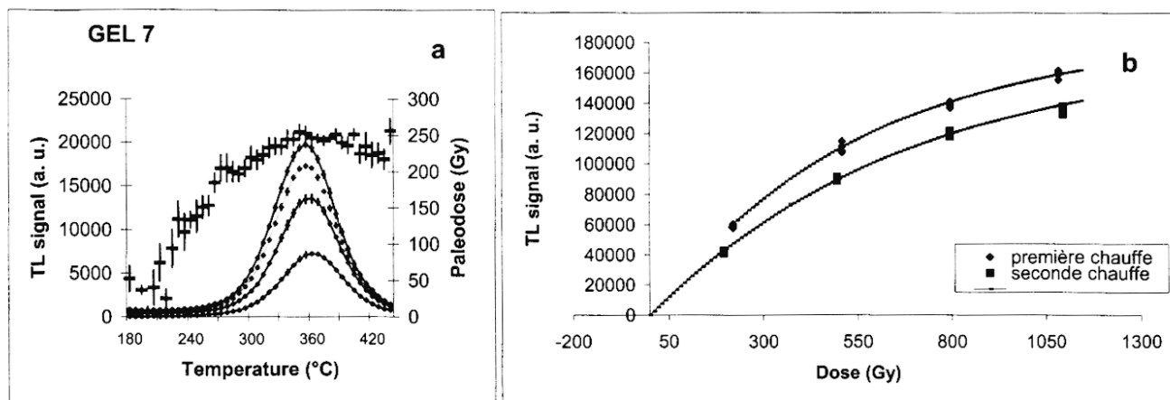
Fig. 6 : Signaux de thermoluminescence de l'échantillon GEL 7. a) Courbes de première chauffe et test du plateau ; b) Courbes de croissance de la TL de première et de seconde chauffe en fonction de la dose accumulée.
