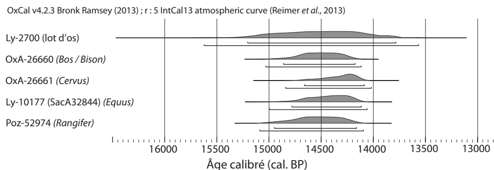
Fig. 2 – Abri Faustin. Courbes de calibration des dates 14 C.
