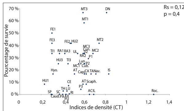
Fig. 5 – Abri Faustin. Diagramme de dispersion des pourcentages de survie en fonction de la densité des éléments (CT). Les abréviations utilisées sont explicitées dans le tableau 5.
