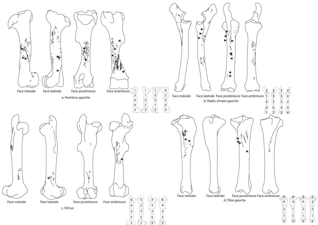
Fig. 13 – Abri Faustin. Localisation des stries et des impacts de percussion sur l'humérus, le radio-ulnaire, le fémur et le tibia. NME par portion anatomique.
