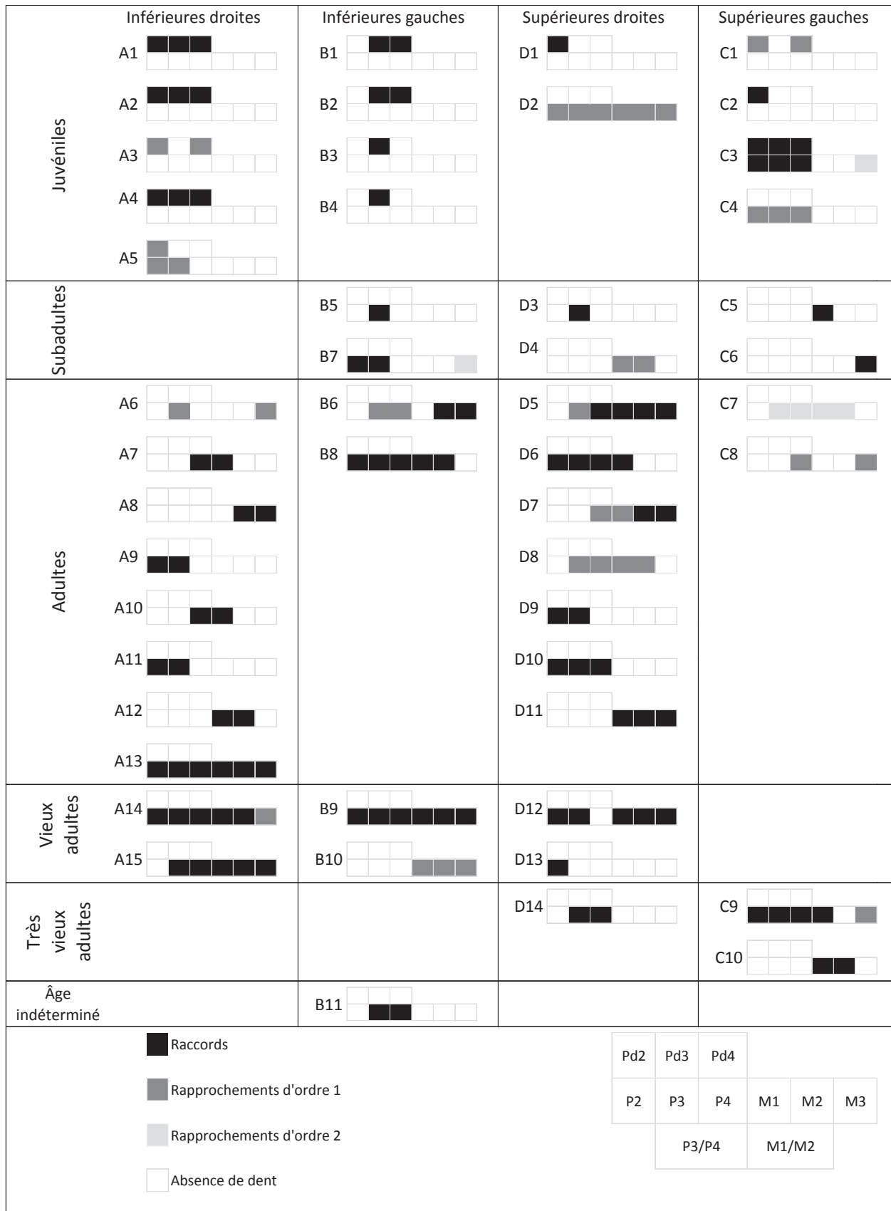
Fig. 8 – Abri Faustin. Répartition des dents des travées 24 et 25 par série. Les séries sont rangées de haut en bas dans l'ordre croissant de maturation dentaire.
