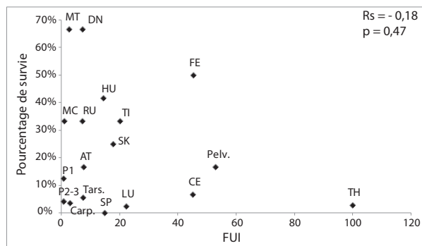
Fig. 6 – Abri Faustin. Diagramme de dispersion des pourcentages de survie en fonction du Food Utility Index (FUI). Les abréviations utilisées sont explicitées dans le tableau 5.
