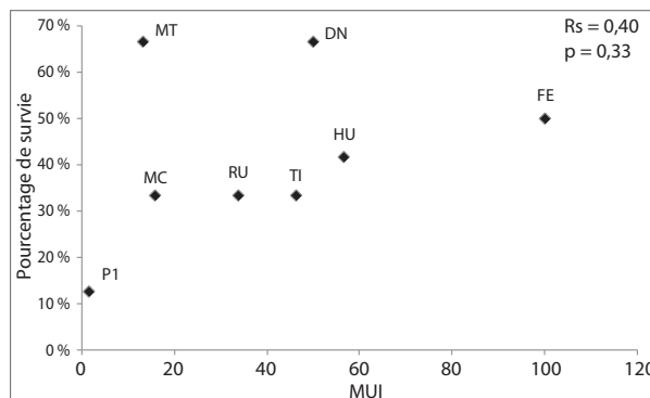
Fig. 7 – Abri Faustin. Diagramme de dispersion des pourcentages de survie en fonction du Marrow Utility Index (MUI). Les abréviations utilisées sont explicitées dans le tableau 5.
