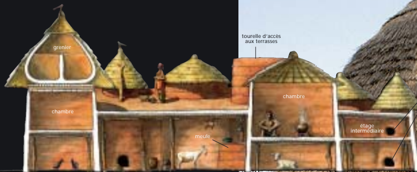
COUPE AA
