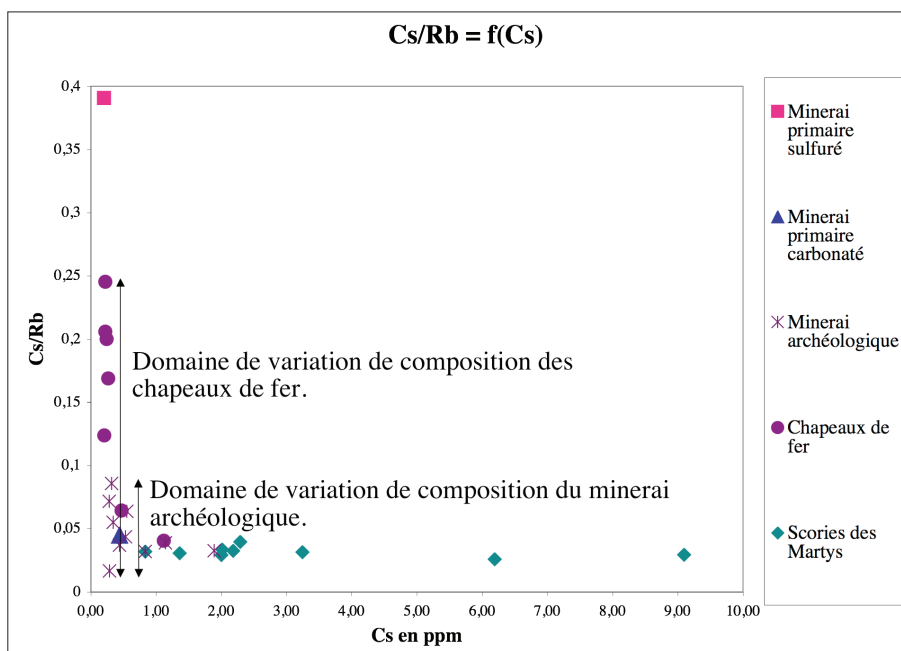
Fig. 2. Variation du rapport Cs/Rb en fonction de la concentration en Cs des différents types de minerais des Martys.
