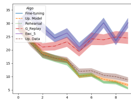
(j) FID VAE
