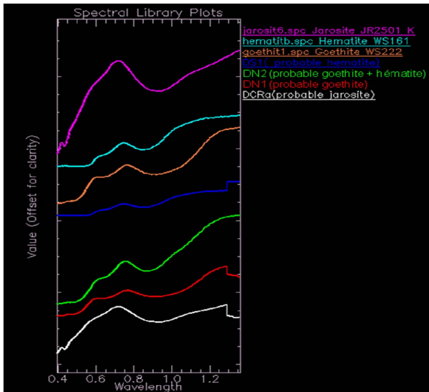
Figure 9 : Comparaison des endmembers probables de la zone minière de Bougrine avec les minéraux purs correspondant dans l'intervalle de spectre qui s'étend de 0,4 à 1,3 \mu\text{m} .
