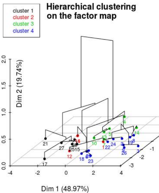
Figure 9 : Classification Hiérarchique
