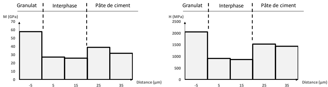
Figure 4. Gradient du module d'indentation et de la dureté au niveau de l'interphase
