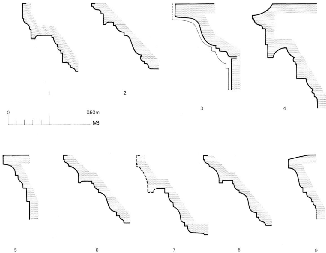
6 Profils comparés de couronnements de podiums (Rome et Gaule Narbonnaise).
