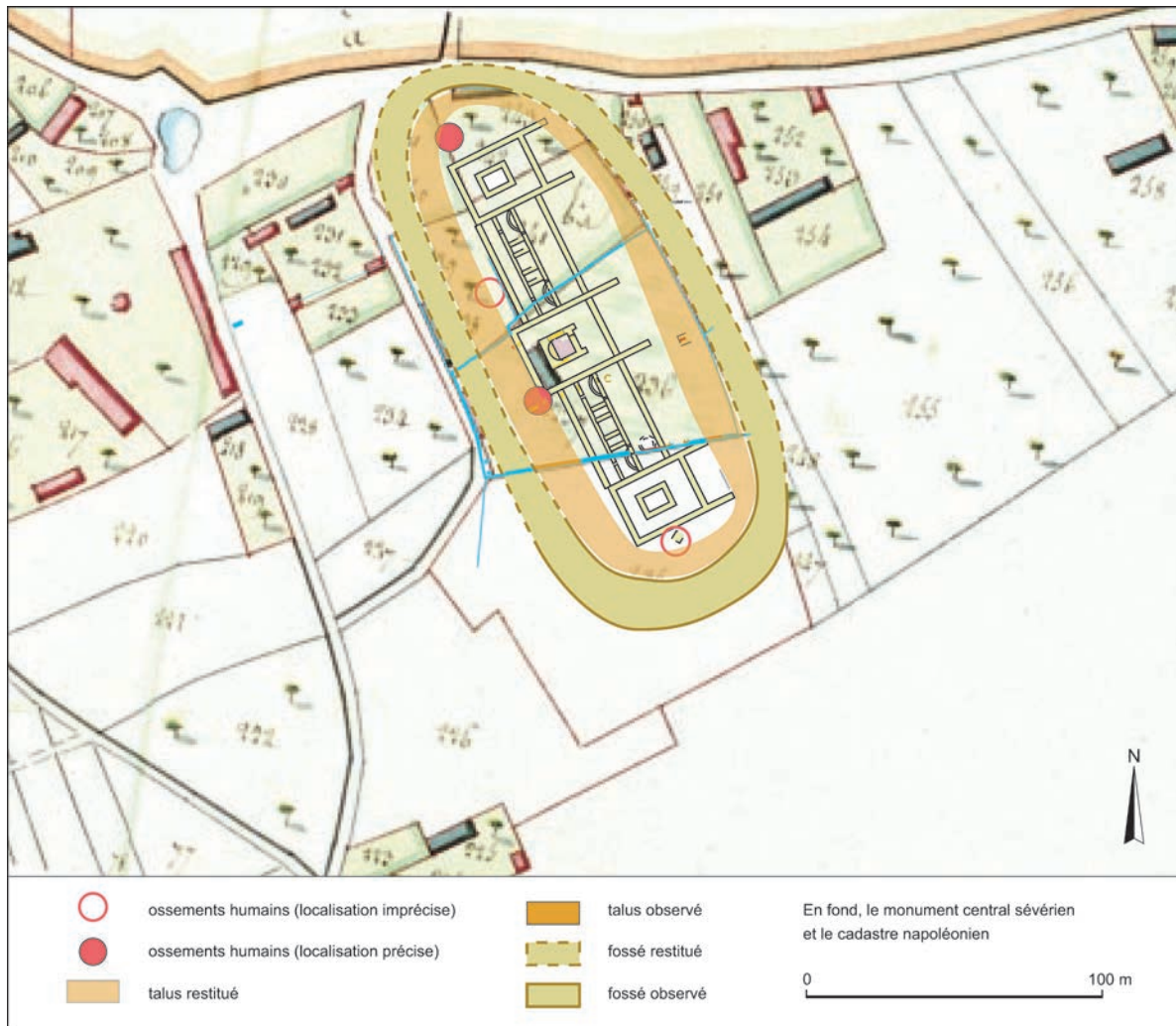
Fig. 34 – Plan général du castellum tardo-antique sur le fond cadastral napoléonien (DAO : L. Guyard, MADE-Département de l'Eure).
