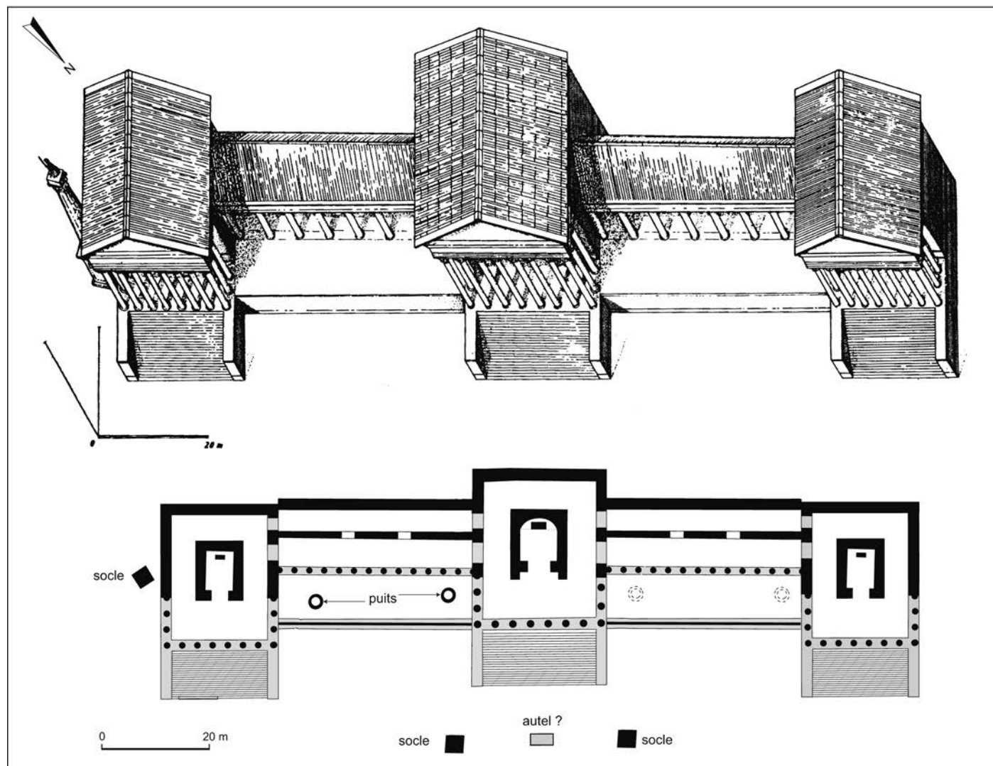
Fig. 30 – Restitution axonométrique des trois temples sévériens du Vieil-Évreux (dessin : V. Brunet ; plan : L. Guyard, MADE-Département de l'Eure).
