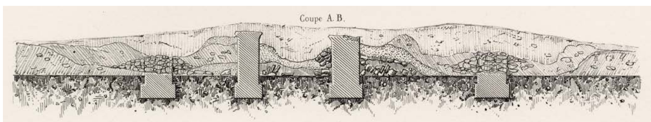
Fig. 36 – Vue de la coupe publiée par Th. Bonnin (d'après Bonnin, 1845, pl. X).
