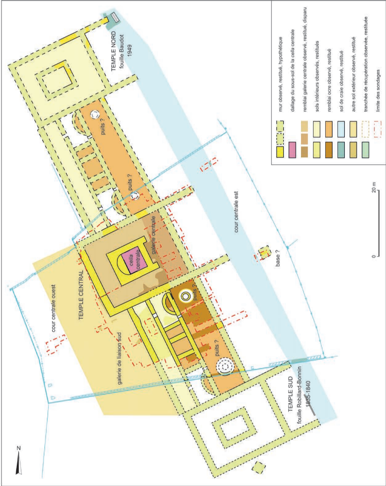
Fig. 29 – Plan de l'état sévérien du grand sanctuaire central du Vieil-Évreux (DAO : L. Guyard et S. Bertaudière, MADE-Département de l'Eure).
