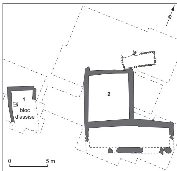
Fig. 136 – Plan de l'établissement rural de la Foucardière à Chênehutte-Trèves-Cunault (Maine-et-Loire) avec, dans le bâtiment 1, un probable bloc d'assise de jumelles (DAO : M. Monteil, Université de Nantes, d'après Boisbouvier, 1980).
