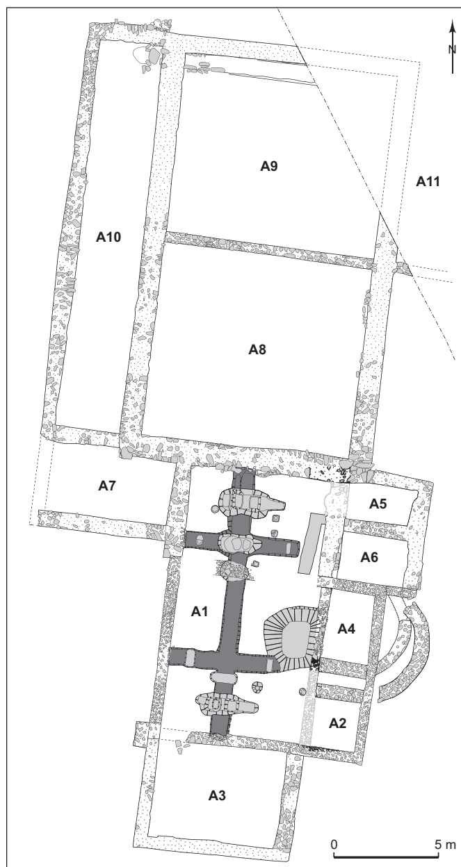
Fig. 116 – Plan du bâtiment A de Piriac-sur-Mer aux I er -III e s. En gris foncé : empreinte du pressoir (DAO : D. Seris et M.-L. Hervé-Monteil, Inrap).
