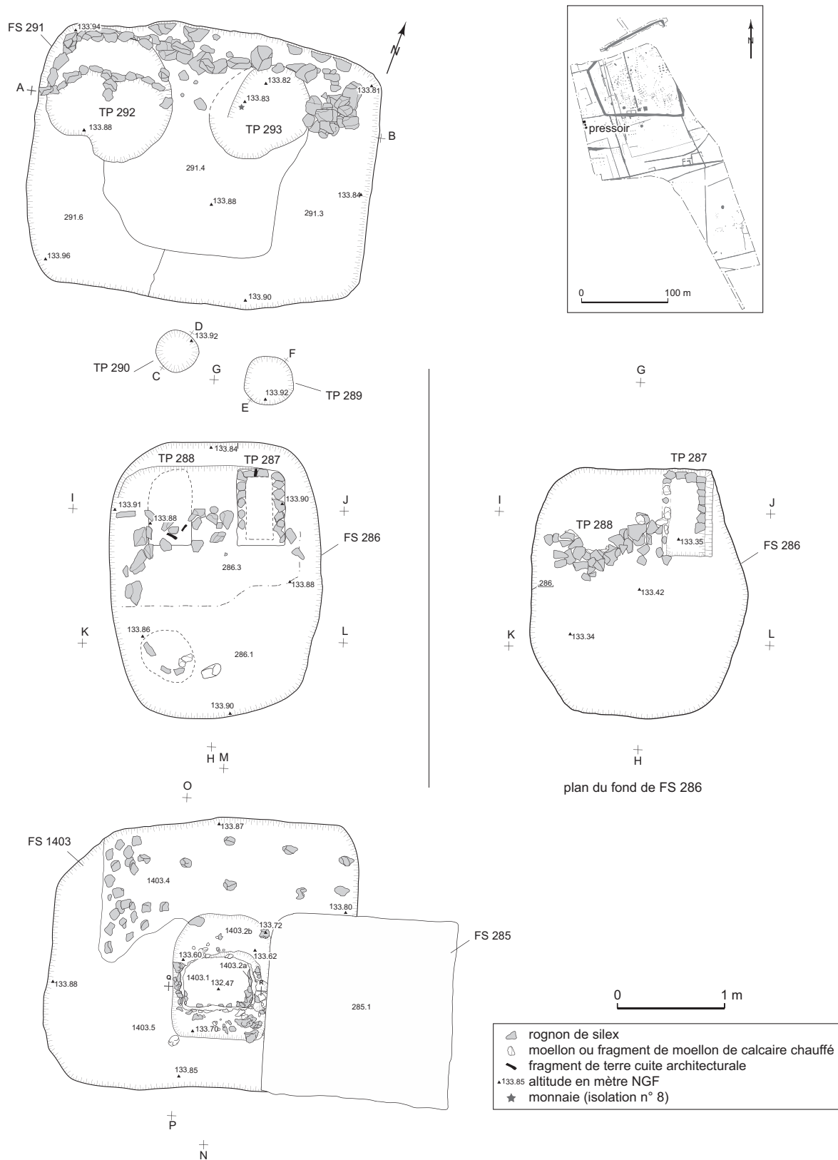
Fig. 104 – Plan du pressoir de Parville (DAO : D. Lépinay et D. Lukas, Inrap).
