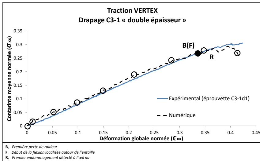
Figure 7 - Courbes Contrainte/Déformation de la plaque composite soumise à de la traction Comparaison numérique/expérimental
