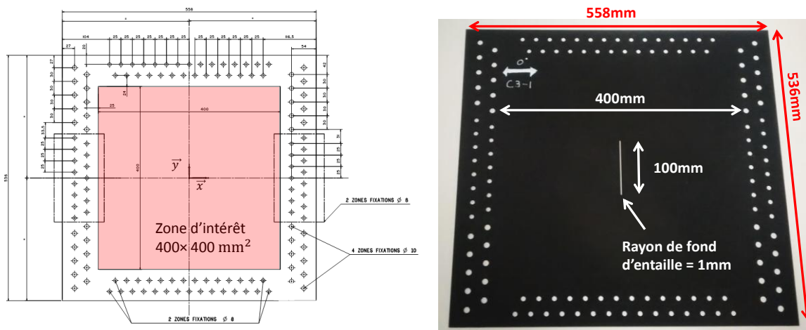
Figure 3 – Partie supérieure du caisson central (à gauche) et Eprouvette composite entaillée (à droite)
