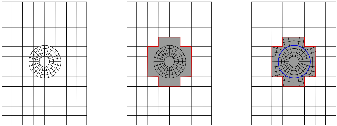
(a) Maillages initiaux (géométries non-conformes). (b) Détermination du patch et de l'interface dans le modèle globale. (c) Maillage de transition faisant apparaître deux interfaces distinctes.
