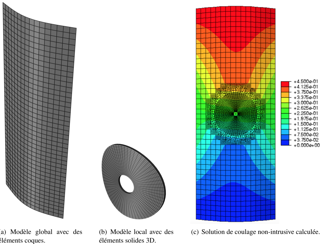
FIGURE 4 – Application de la stratégie développée pour enrichir localement une coque cylindrique.
