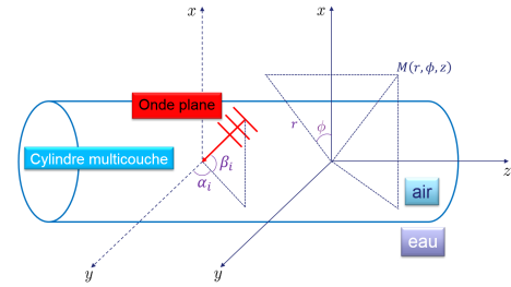
FIGURE 1 – Géométrie de la structure multicouche
