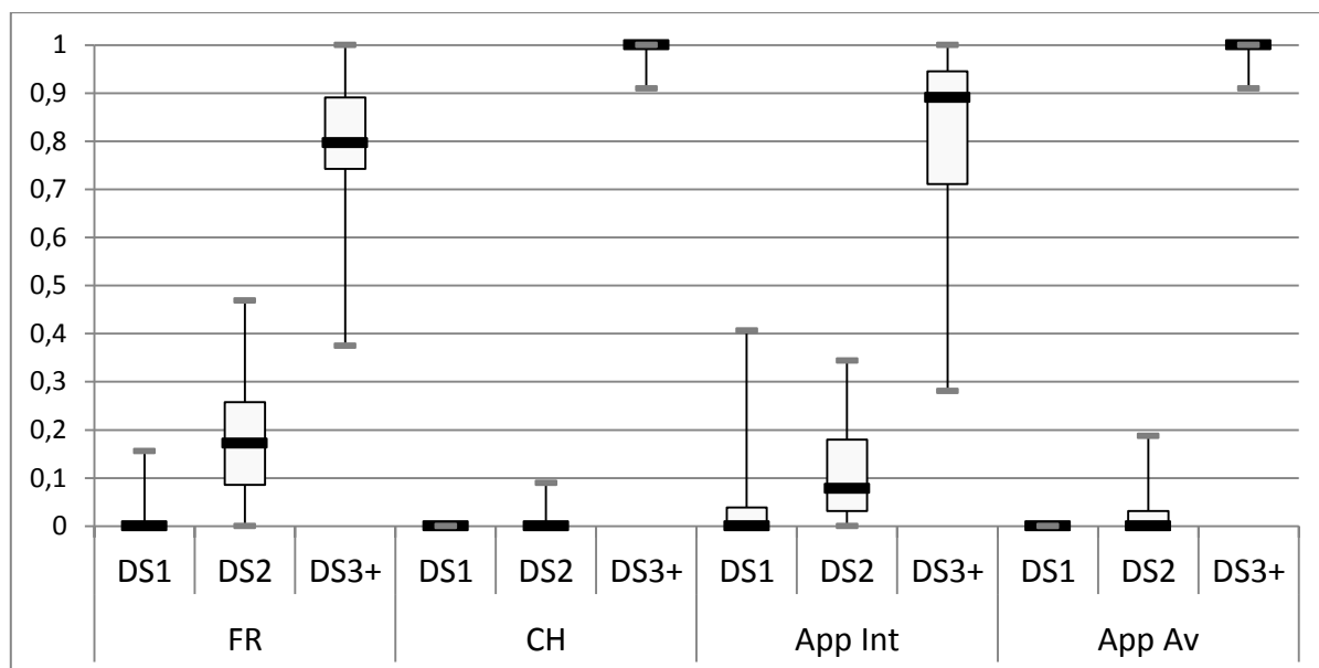
Figure 3. Densité sémantique
