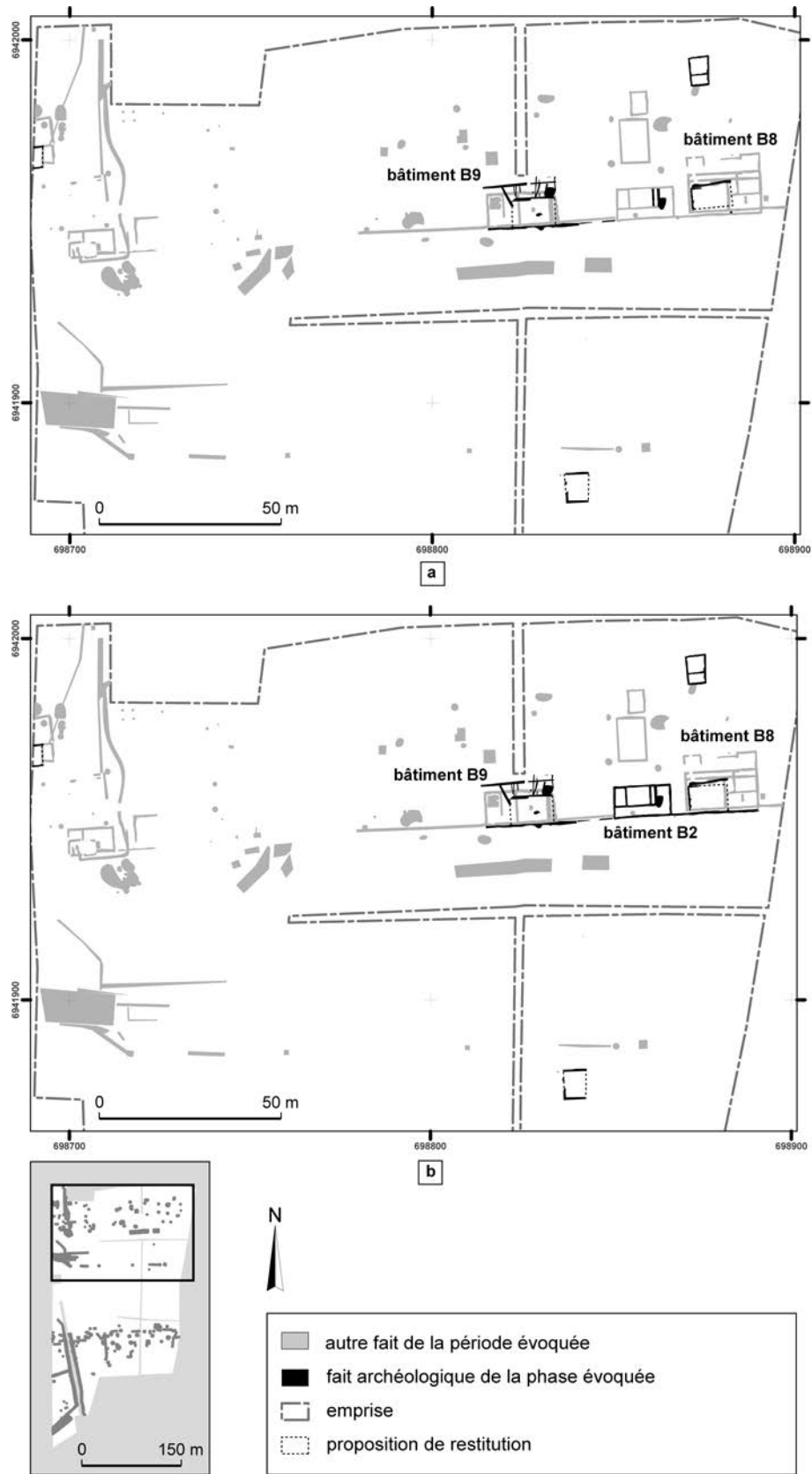
Fig. 7 – Les bâtiments de l'aile nord et de la cour : a, état 2, phase 1 ; b, état 2, phase 2 (DAO : C. Font, Inrap).
