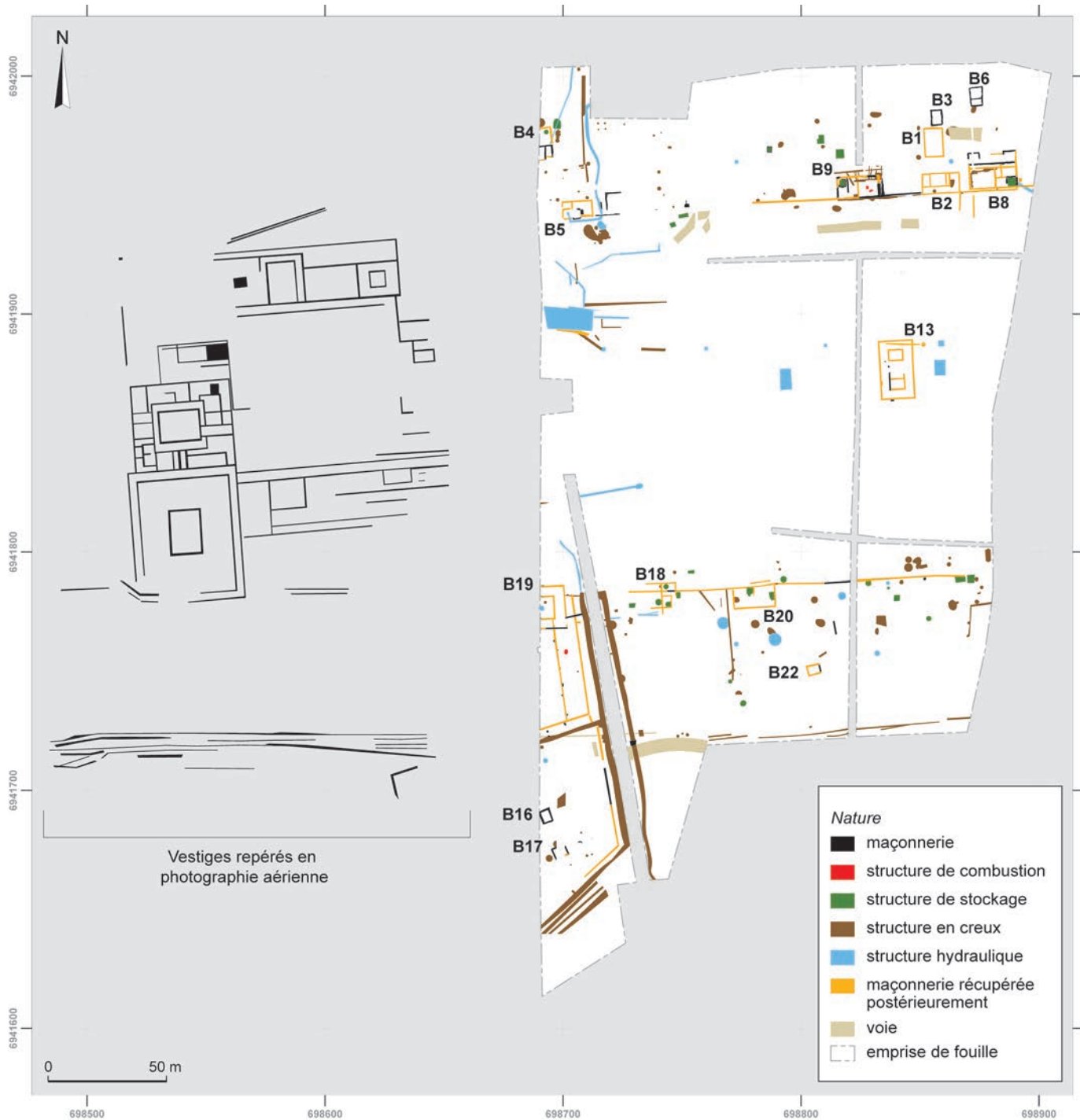
Fig. 6 – Plan du deuxième état du site (d'après le cliché de A. Normier, Des ailes pour la science ; topographie et photo-redressement : A. Bolo, Inrap ; DAO : C. Font, Inrap).
