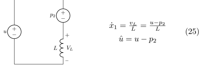
Fig. 4. Parameter p_2 to estimate \hat{u}
