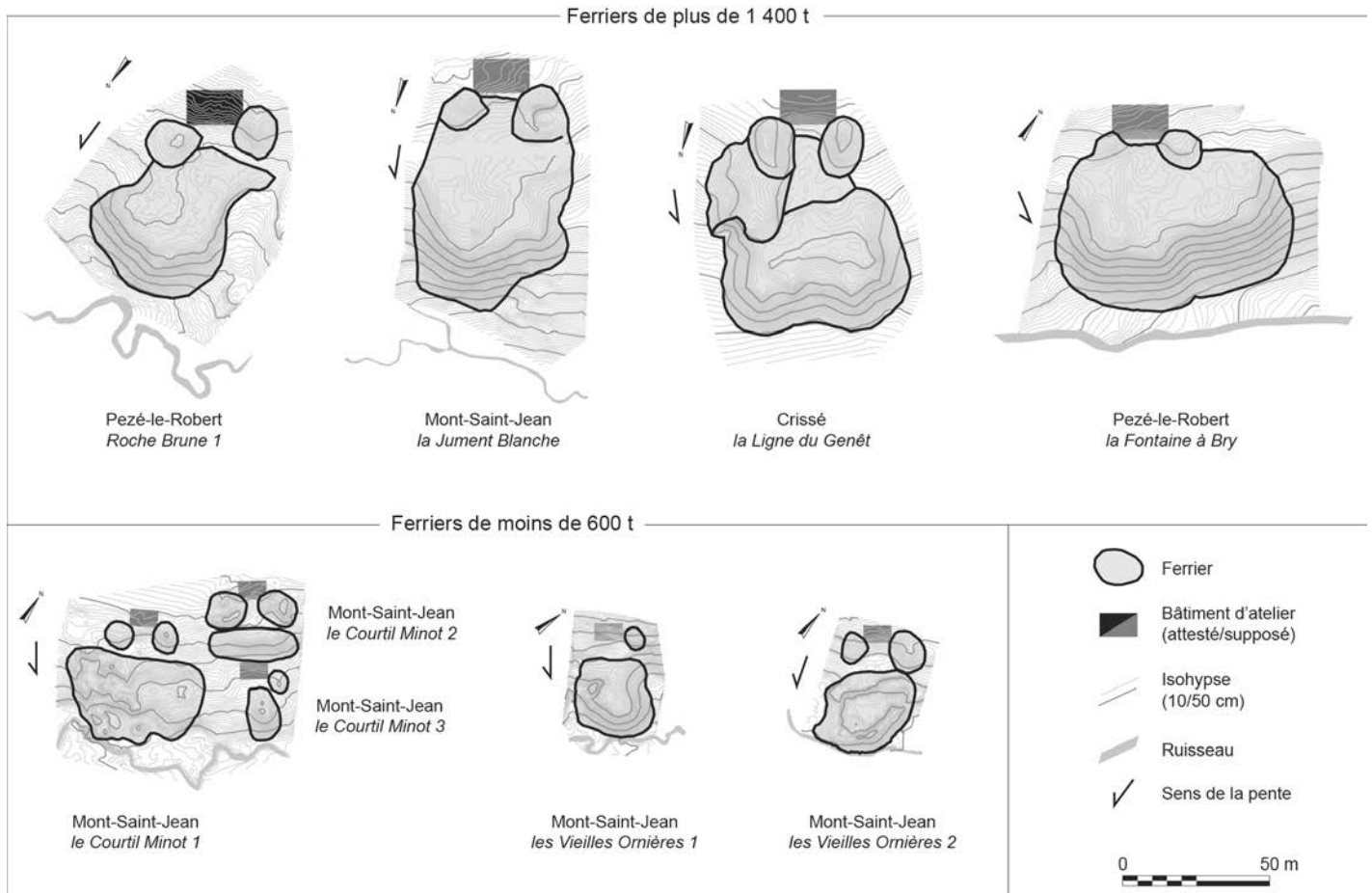
Fig. 3 – Plans simplifiés des sites de réduction directe ayant fait l'objet d'un relevé topographique. Deux groupes se différencient : les grands ferriers, de plus de 1400 t, et les petits, de moins de 600 t (DAO : F. Sarreste, CAPRA/Éveha).
