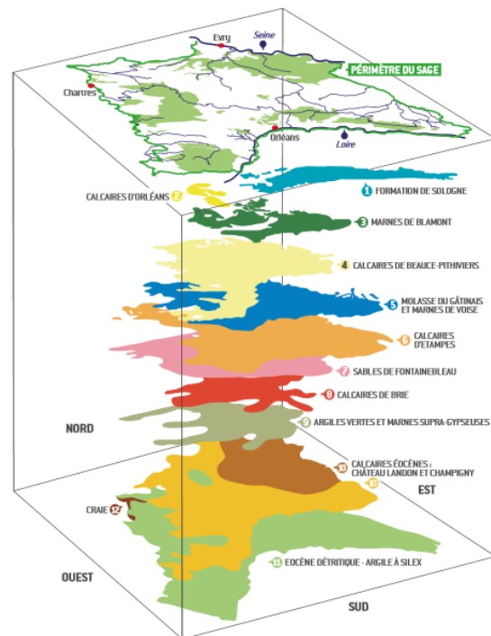
Figure 19: Esquisse géologique de la nappe de Beauce.
