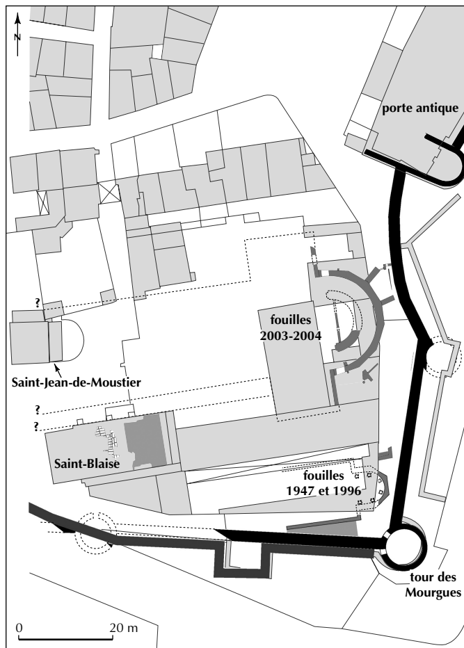
Fig. 59 – Arles (Bouches-du-Rhône). Église de l'enclos Saint-Césaire : plan restitué de l'église dans son environnement (DAO M. Heijmans, CNRS).
