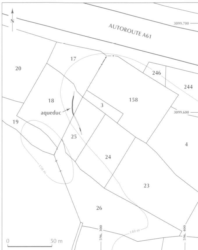
Fig. 98 – Localisation topographique et cadastrale de l'aqueduc de Sur Fontorbe à Lavalette et Carcassonne (DAO M. Passelac, CNRS).
