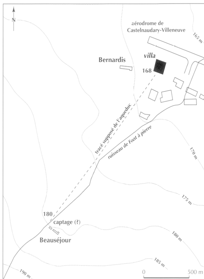
Fig. 109 – Mas-Saintes-Puelles, aqueduc de La Baronne et villa de Bernardis dans leur contexte topographique et hydrographique (DAO M. Passelac, CNRS).
