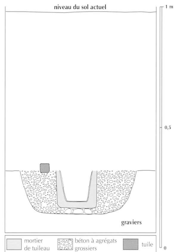
Fig. 105 – Bartissol à Castelnaudary : section dans le fossé de la parcelle 76 de l'aqueduc (DAO M. Passelac, CNRS).
