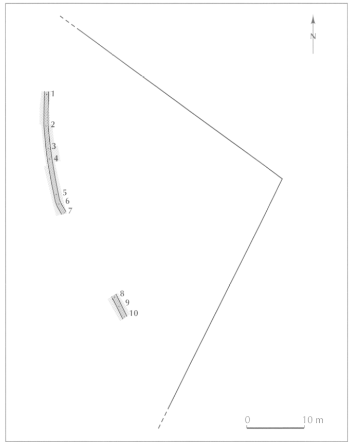
Fig. 99 – Sur Fontorbe à Lavalette et Carcassonne : plan du chantier et localisation des points d'observation et de mesures (DAO M. Passelac, CNRS).
