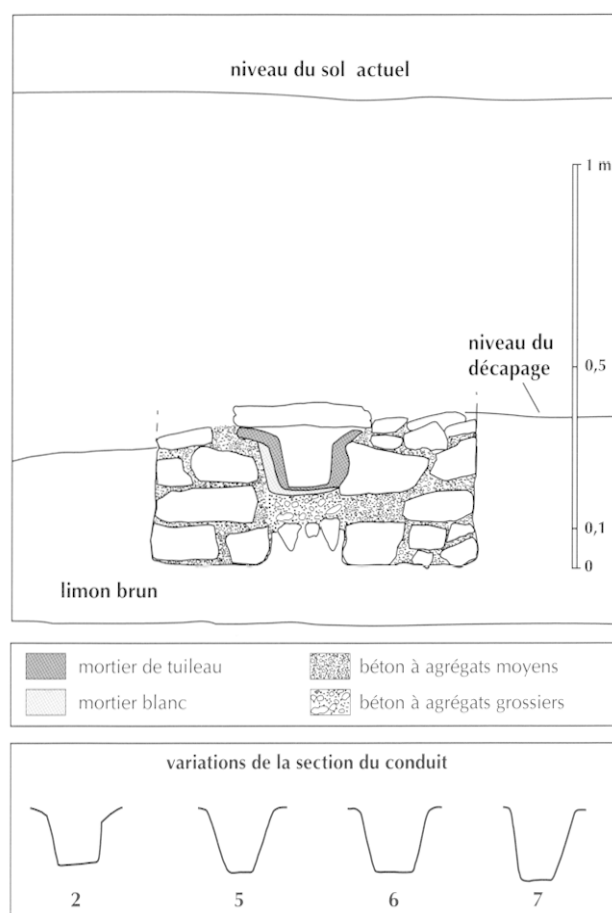
Fig. 101 – Sur Fontorbe à Lavalette et Carcassonne : section de l'aqueduc au point 2 et variations de la section du conduit (DAO M. Passelac, CNRS).
