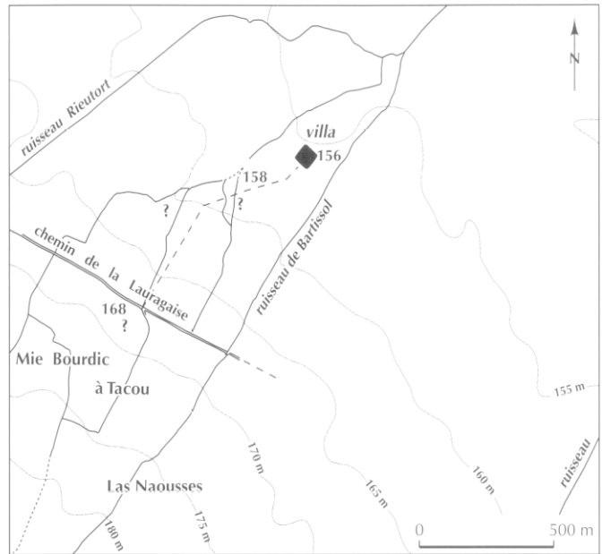
Fig. 106 – Bartissol à Castelnaudary : contexte topographique et hydrographique de l'aqueduc, d'après le cadastre de 1823 (DAO M. Passelac, CNRS).
