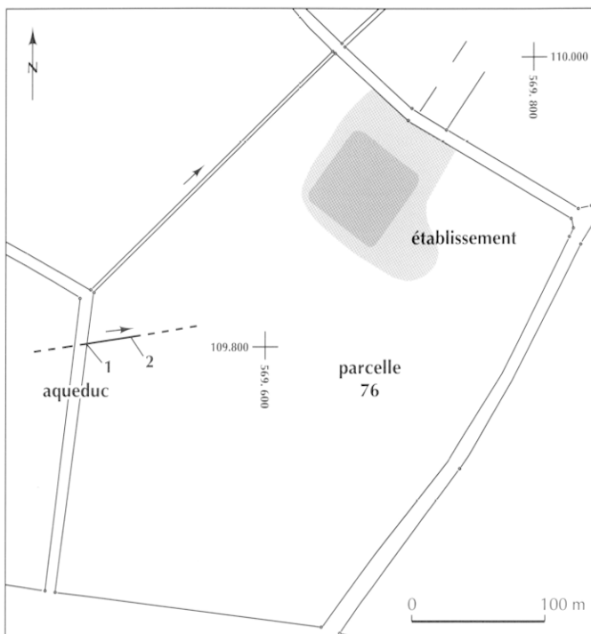
Fig. 104 – Bartissol à Castelnaudary : localisation cadastrale de l'aqueduc et de l'établissement rural (DAO M. Passelac, CNRS).
