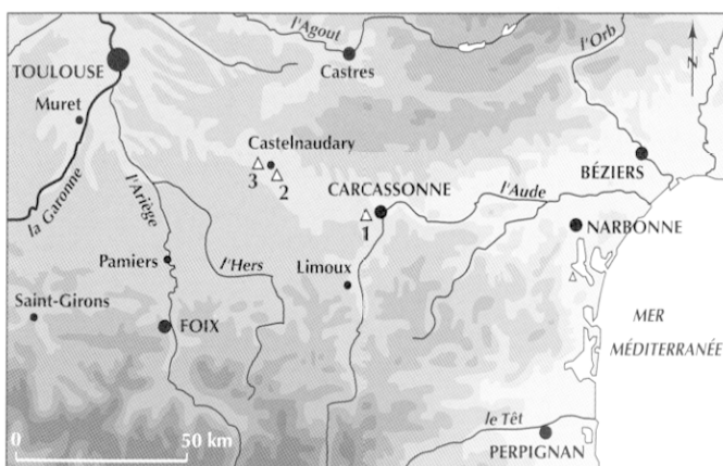
Fig. 97 – Localisation des sites étudiés dans le bassin occidental de l'Aude : 1, Sur Fontorbe à Lavalette et Carcassonne ; 2, Bartissol à Castelnaudary ; 3, La Baronne à Mas-Saintes-Puelles (DAO M. Passelac, CNRS).
