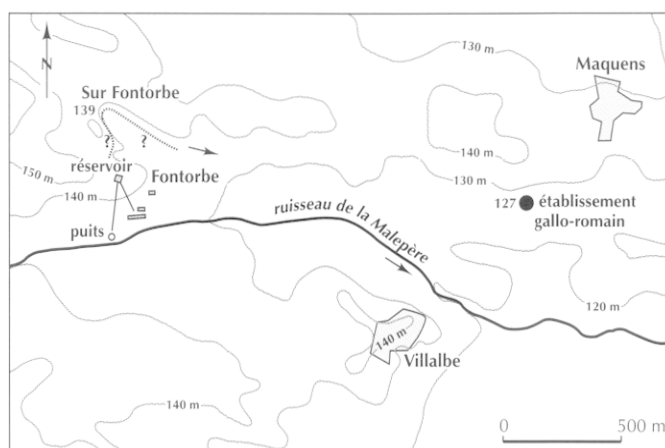
Fig. 103 – Sur Fontorbe à Lavalette et Carcassonne : contexte topographique et hydrographique de l'aqueduc (DAO M. Passelac, CNRS).
