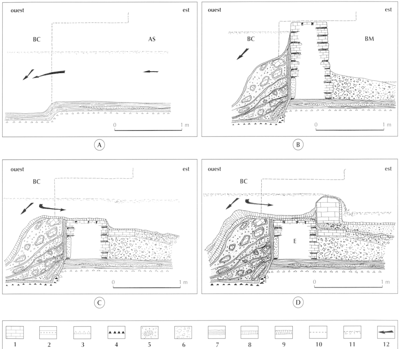
Fig. 84 – Coupes de l'évolution dans le temps des dépôts et du fonctionnement de l'aqueduc au niveau du mur occidental du bras mort (voir fig. 80, n° 5) : A, première phase, convergence des aqueducs nord et sud, dépôt des concrétions de première génération (I er s. ?) ; B, deuxième phase, restauration du bassin de convergence et séparation des aqueducs nord et sud (II e s. ?), dépôt des concrétions de deuxième génération ; C, troisième phase, abaissement du mur occidental du bras mort et réutilisation de l'ex-bras mort pour dériver une partie des eaux de l'aqueduc nord vers les moulins de Barbegal via l'aqueduc sud, dépôt des concrétions de troisième génération ; D, quatrième phase, édification de l'étranglement du bras mort (seuil pour réguler le débit ?) (voir fig. 80, n° 4), dépôt des concrétions de quatrième génération ; 1, blocs de calcaire de l'édifice ou remaniés ; 2, tuiles ou briques ; 3, enduit de mortier de tuileau de première génération ; 4, enduit de mortier de tuileau de deuxième génération ; 5, dépôts détritiques à éléments roulés et encroûtés ; 6, formations détritiques à éléments anguleux (débris de taille essentiellement) ; 7, ensemble concrétionné de première génération ; 8, ensemble concrétionné de deuxième génération ; 9, ensemble concrétionné de troisième et quatrième générations ; 10, silhouette du bâti situé au second plan ; 11, niveau moyen de l'eau dans l'ouvrage ; 12, sens de l'écoulement des eaux ; BC, bassin de convergence ; AS, aqueduc sud ; BM, bras mort ; E, étranglement du bras mort (dessin J.-L. Guendon, CNRS ; DAO G. Drouiller, CNRS).
