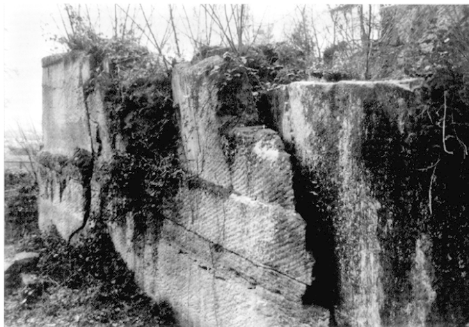
Fig. 123 – Lithoclasé parcourant la carrière du Kriemhildenstuhl (Bad Dürkheim) en direction nord-ouest/sud-est et marquant la limite entre plusieurs secteurs de travail (photo P. Adam).
