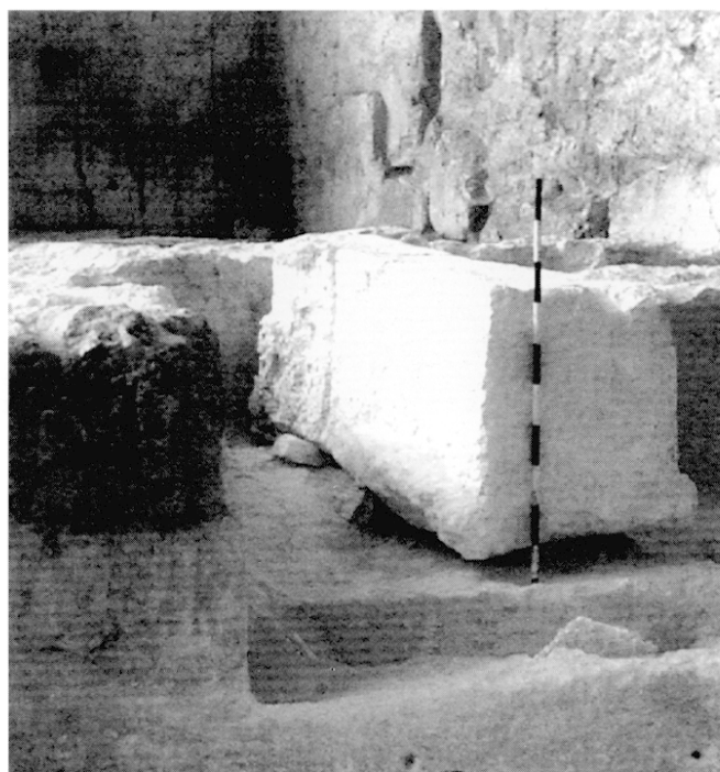
Fig. 75 – Grand bloc basculé hors de son gîte, mis en chantier sur des cales en pierre et abandonné en cours de traitement (dégrossissage de la face d'arrachement et morcellement) (photo G. Monthel, CNRS).
