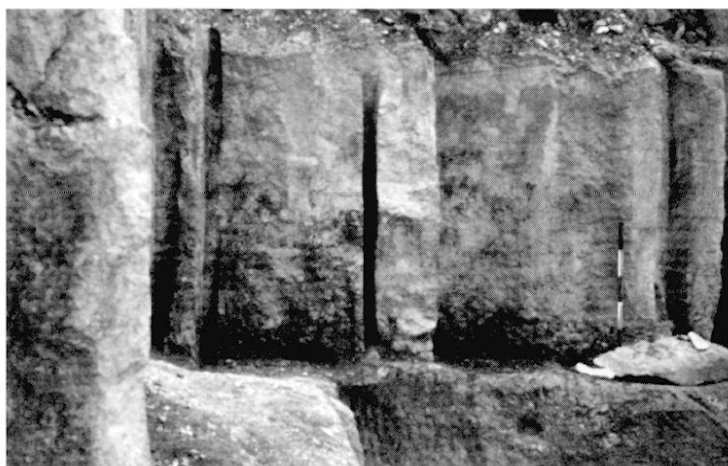
Fig. 70 – Technique pratiquée à l'ouest de la carrière pour les enlèvements verticaux (photo et dessin G. Monthel, CNRS).
