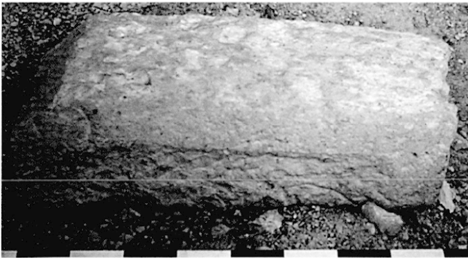
Fig. 76 – Bloc muni de son cadre et de son démaigrissement d'anathyrose. Son arête vive, à gauche, est abattue car peut-être destinée à recevoir une modénature après sa mise en œuvre (photo G. Montheil, CNRS).
