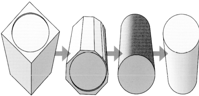
Fig. 78 – Étapes de taillage d'un fût de colonne : 1, levage vertical d'un bloc de plan carré et d'une hauteur égale à celle désirée pour le fût, marqué à chaque extrémité d'un cercle épannelé donnant approximativement le diamètre de ce fût ; 2, épannelage par plans successifs de plus en plus serrés pour obtenir un cylindre dont le diamètre est réglé sur les cercles des extrémités ; 3, épannelage fin du cylindre ; 4, égrissage et polissage réalisés au tour (dessin G. Monthel).
