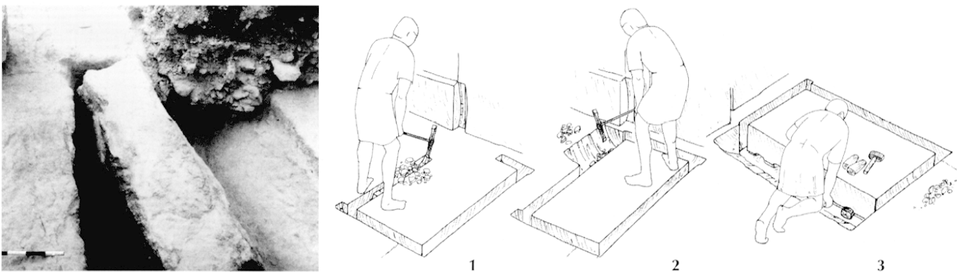
Fig. 64 – Bloc de défermage abandonné in situ et reconstitution des étapes de son enlèvement (dessin et photo G. Monthel, CNRS).
