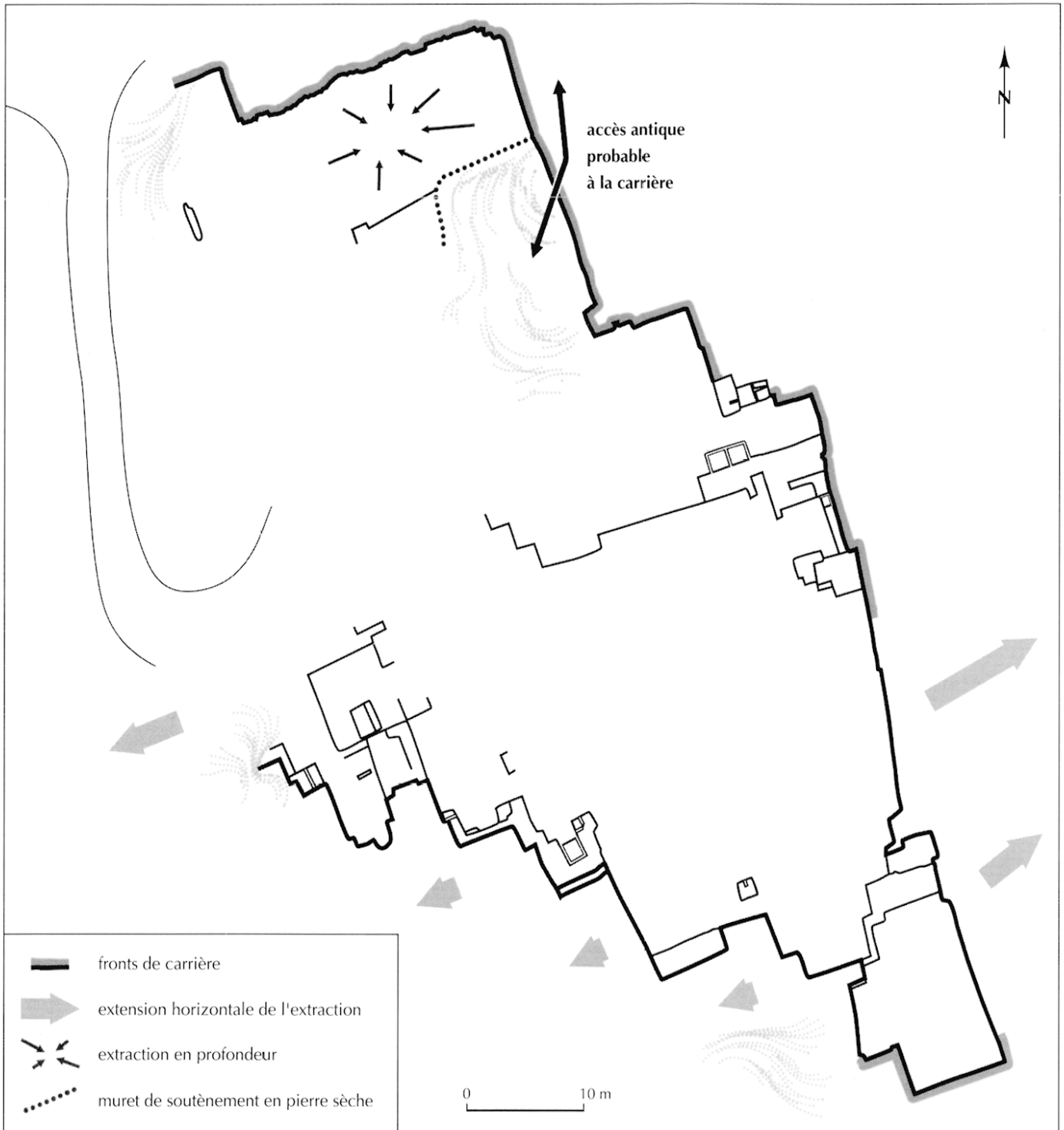
Fig. 61 – Plan de la carrière découverte en 1971 (dessin G. Monthel, CNRS).
