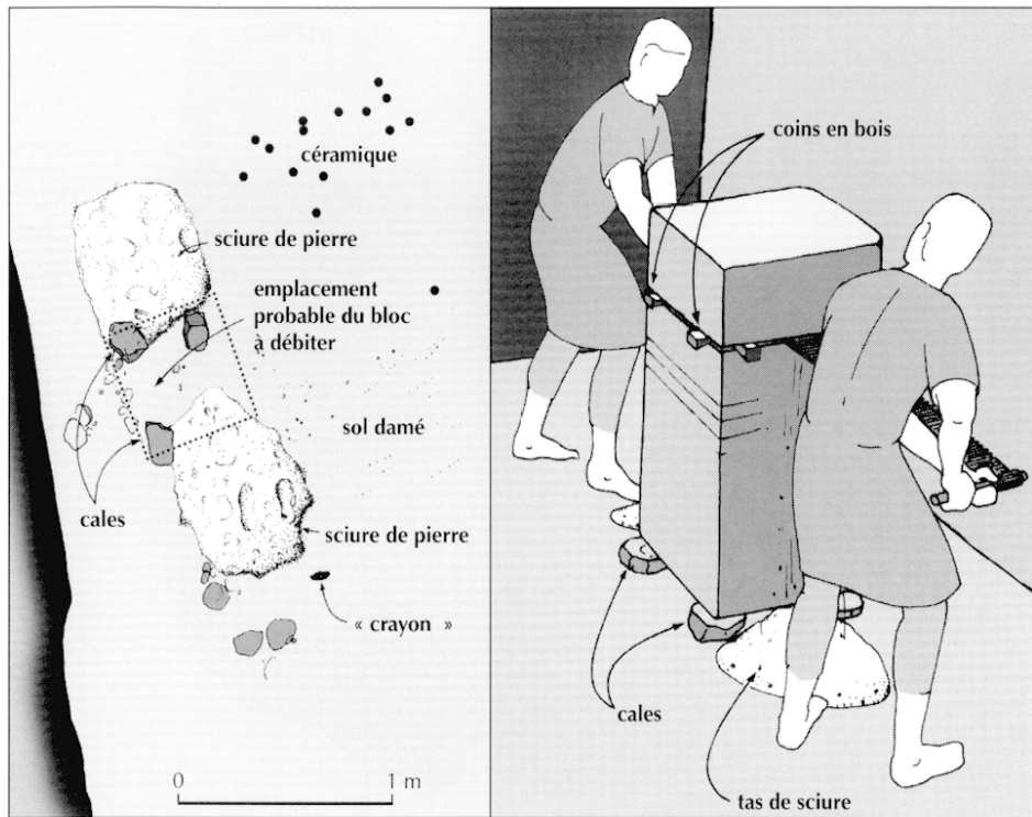
Fig. 77 – Atelier de sciage en sous-main situé à l'ouest de la carrière. Plan et restitution probable (dessin G. Monthel, CNRS).
