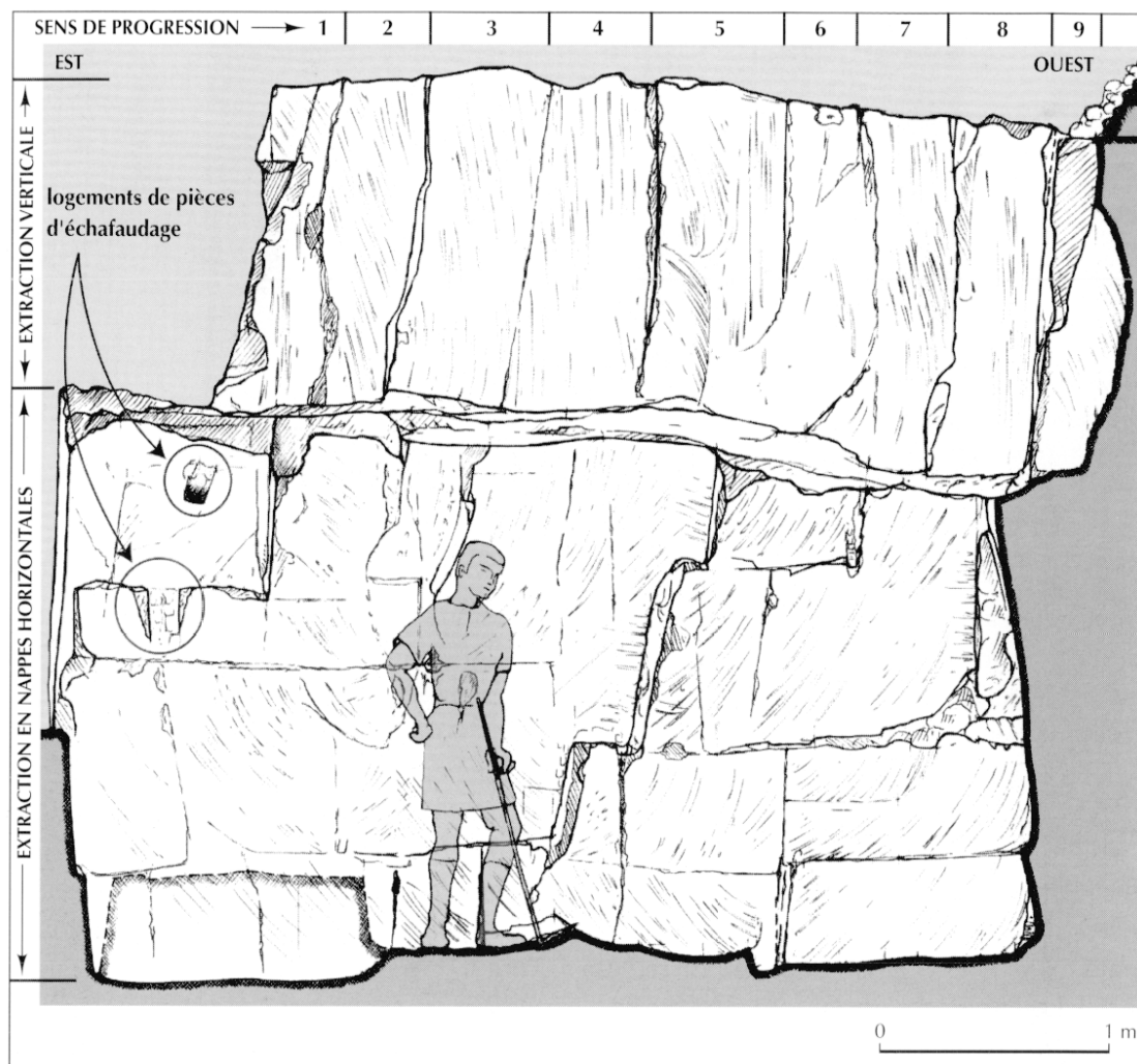
Fig. 71 – Élévation sud des fronts à l'ouest de la carrière. Celle-ci montre les différences de traitement de la paroi entre les enlèvements verticaux par reprise, en haut, et les enlèvements par nappes horizontales qui les ont précédés, en bas (dessin G. Monthel, CNRS).
