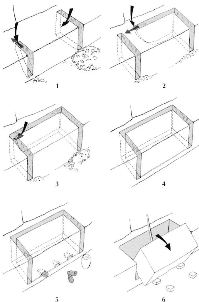
Fig. 65 – Reconstitution des étapes d'extraction d'un bloc (dessin G. Monthel, CNRS).
